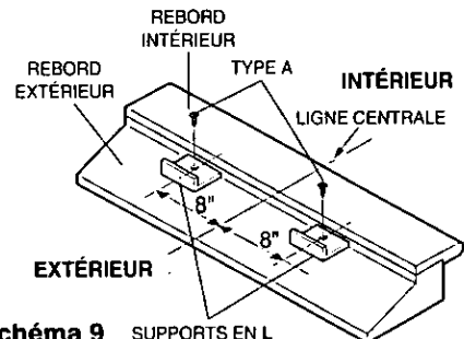
Schéma 9 SUPPORTS EN L
